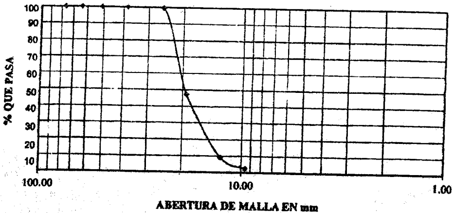
CURVA GRANULOMETRICA
